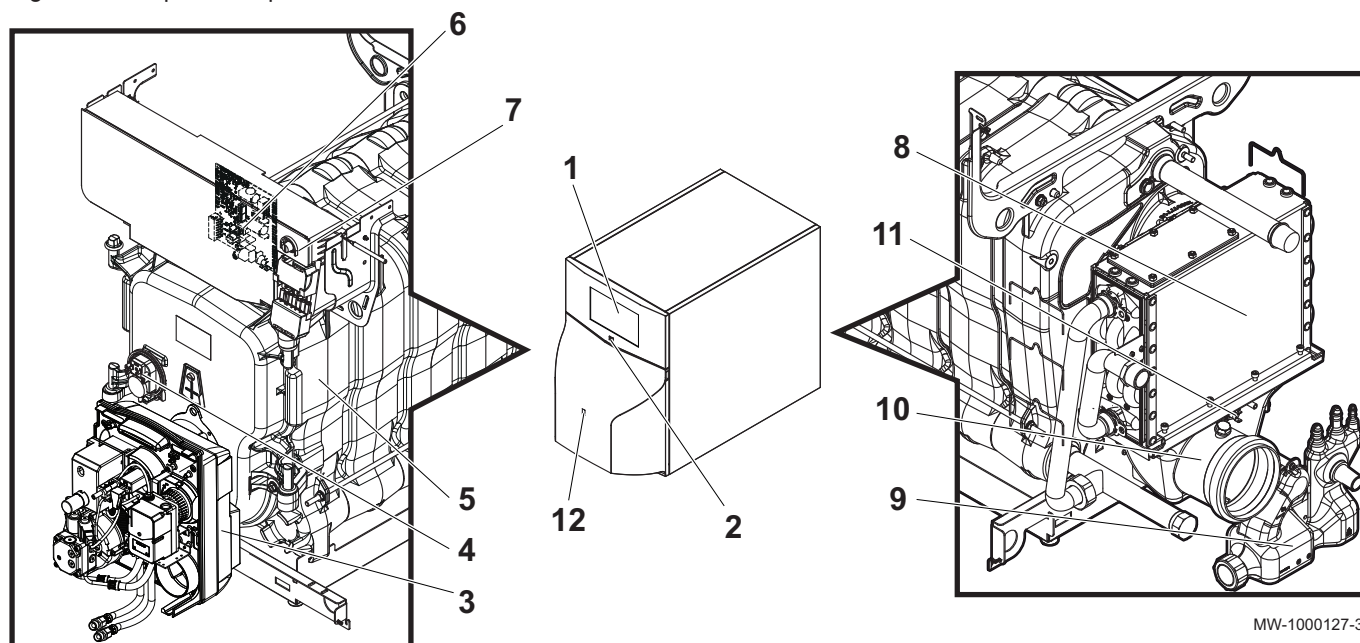
Fig.2 Principaux composants
