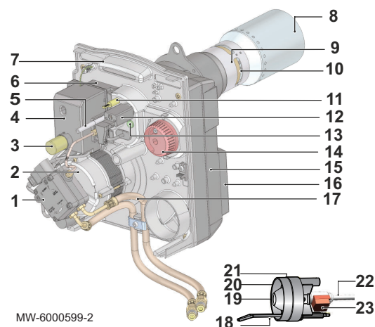
Fig.3 Principaux composants
